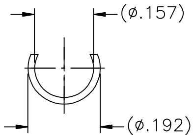
SECTION "A-A" SCALE: 4X
