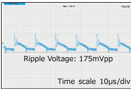
V_{IN}=100Vac, I_{OUT}=1.0A
