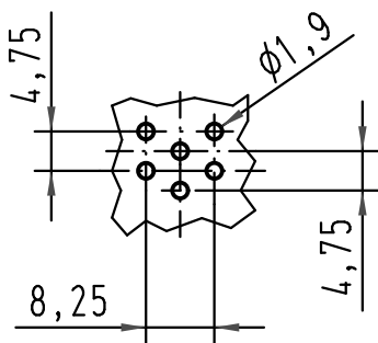
Lochbild / pinhole pattern
