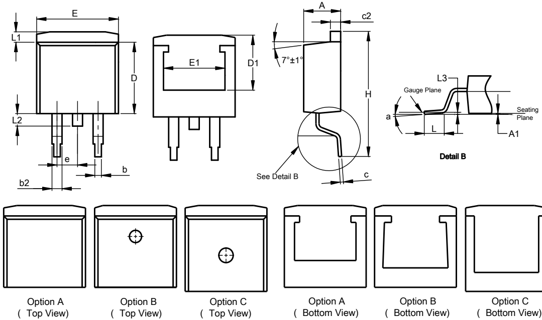
TO263AB (Standard)
