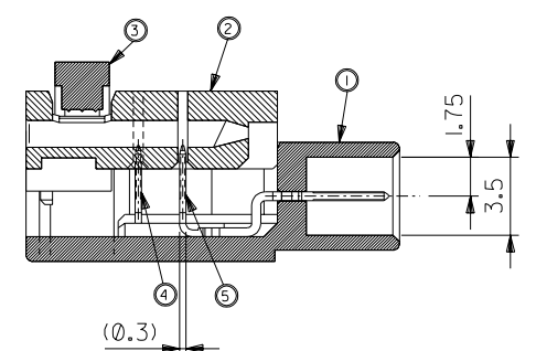
SECT A-A
