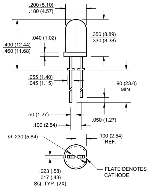
HLMP-D155A
